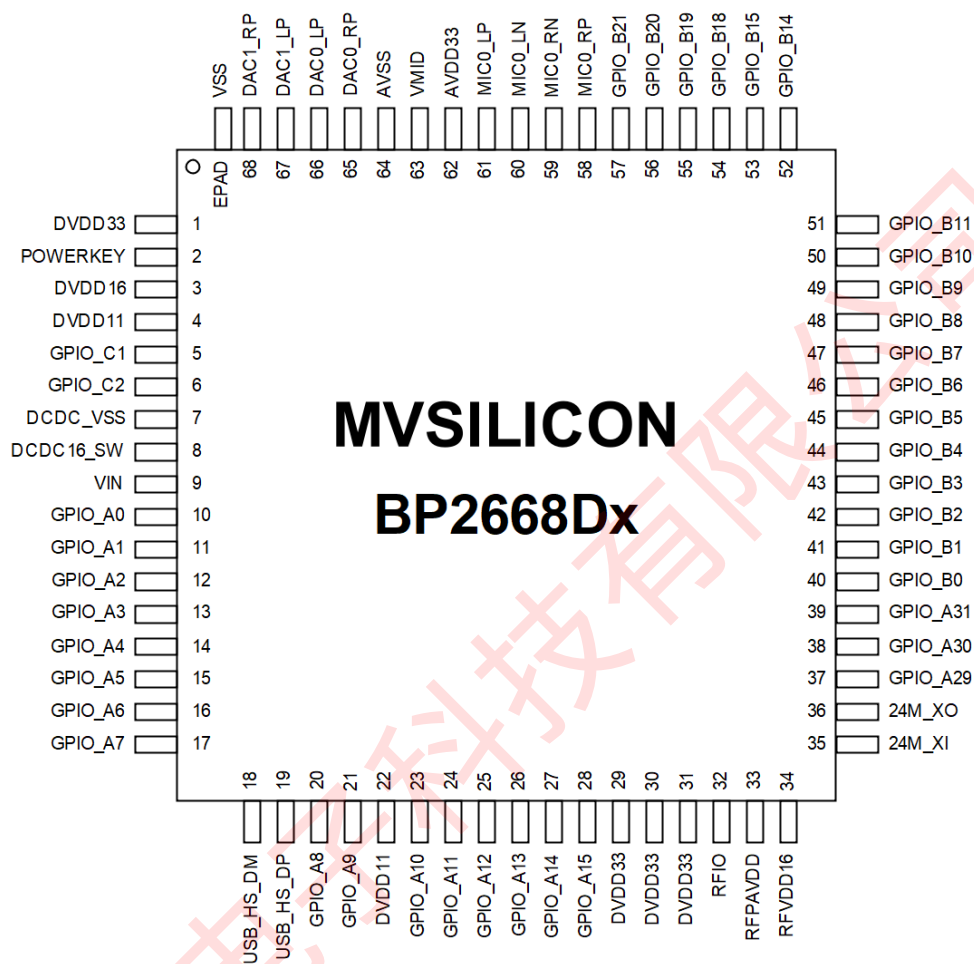
图 2. 芯片引脚定义
